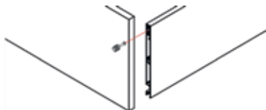
Stabilisateur façade pour tiroirs Vionaro avec hauteur 185 mm
