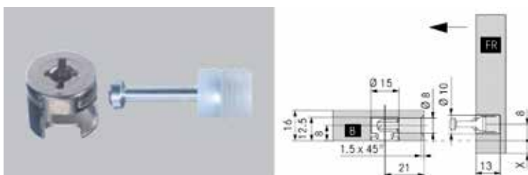
Raidisseur pour tiroirs pour Scala - pour façades avec largeur > 800 mm
