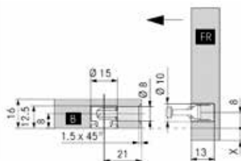
Raidisseur pour tiroirs pour Scala
