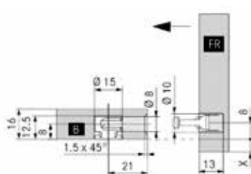
Raidisseur pour tiroirs pour Scala - pour façades avec largeur > 800 mm
